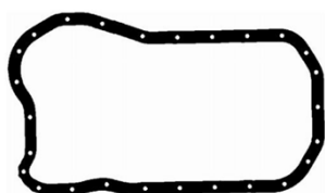
50007 Jta do Carter
