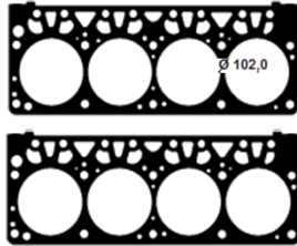
GJ 053 Junta do Cabeçote
