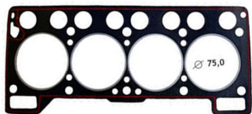
GJ 135 Junta do Cabeçote
