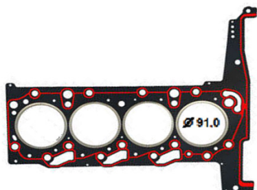
GJ 057 Junta do Cabeçote
