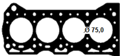
GJ 082 Junta do Cabeçote
