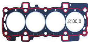
11200170 Junta do Cabeçote
