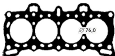
GJ 075 Junta do Cabeçote
