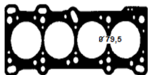
GJ 087 Junta do Cabeçote
