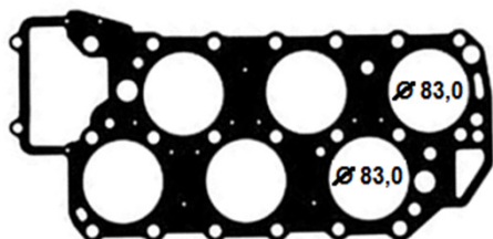
GJ 147 Junta do Cabeçote
